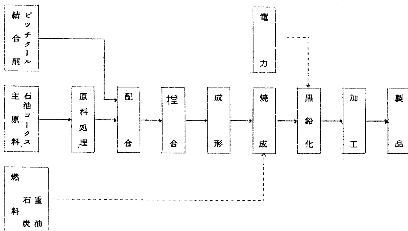
人 造 黒 鉛 電 極 製 造 工 程 図
