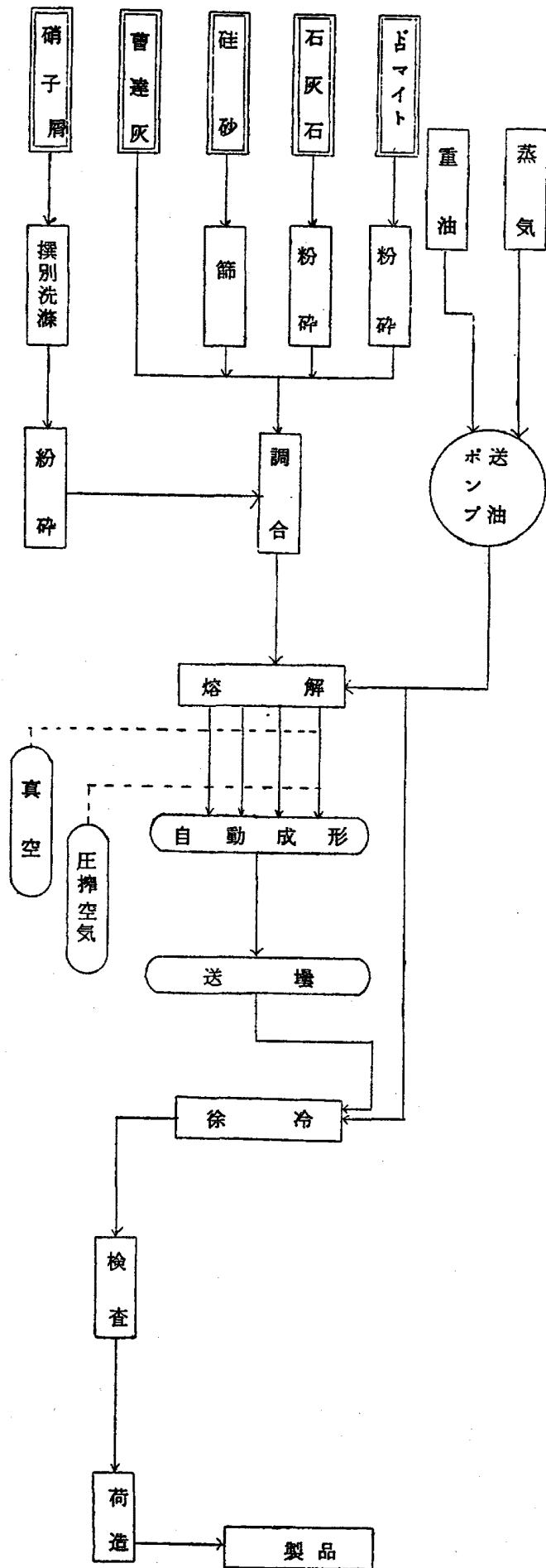
壙製造工程図
