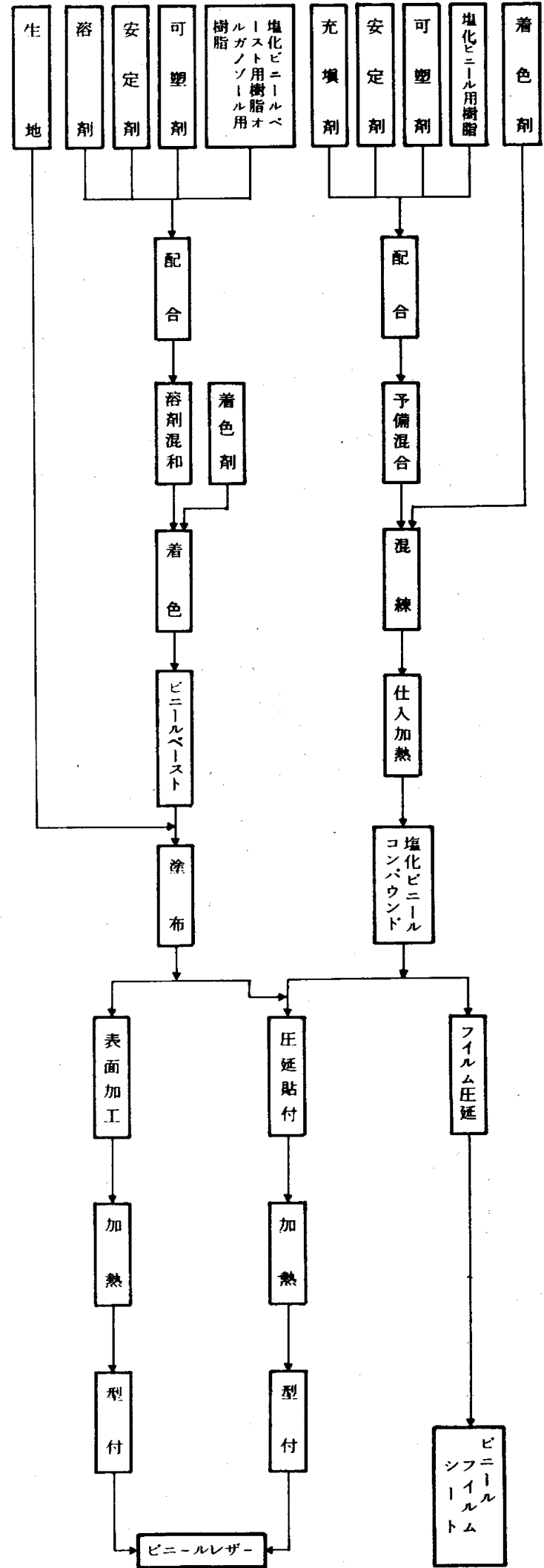
ビニール製品製造工程図
