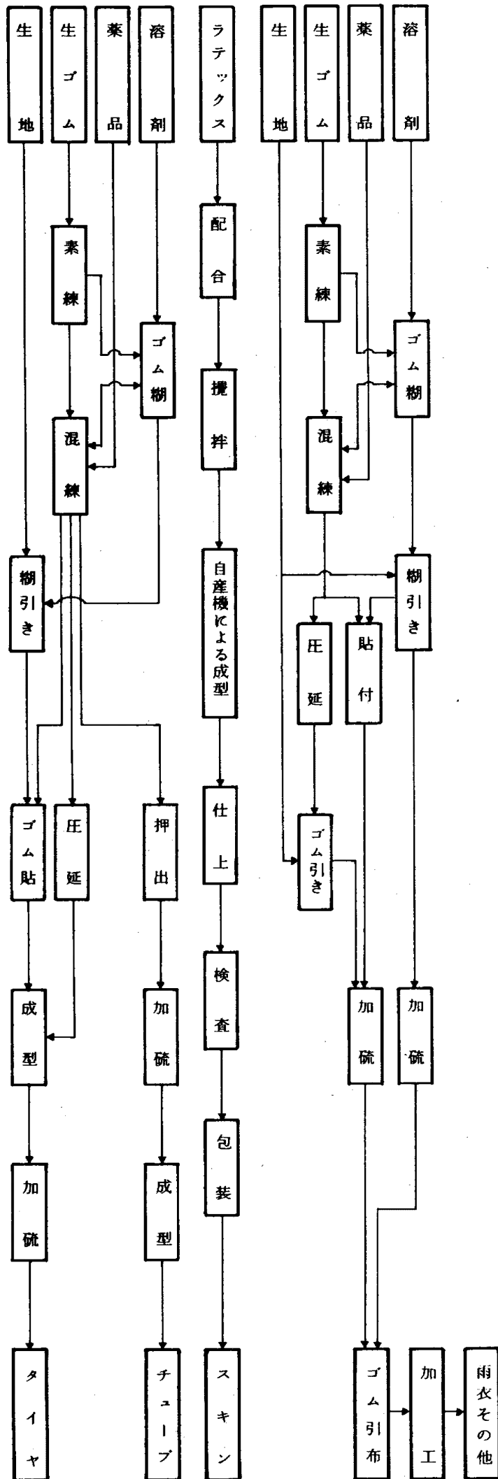
ゴム製品製造工程図
