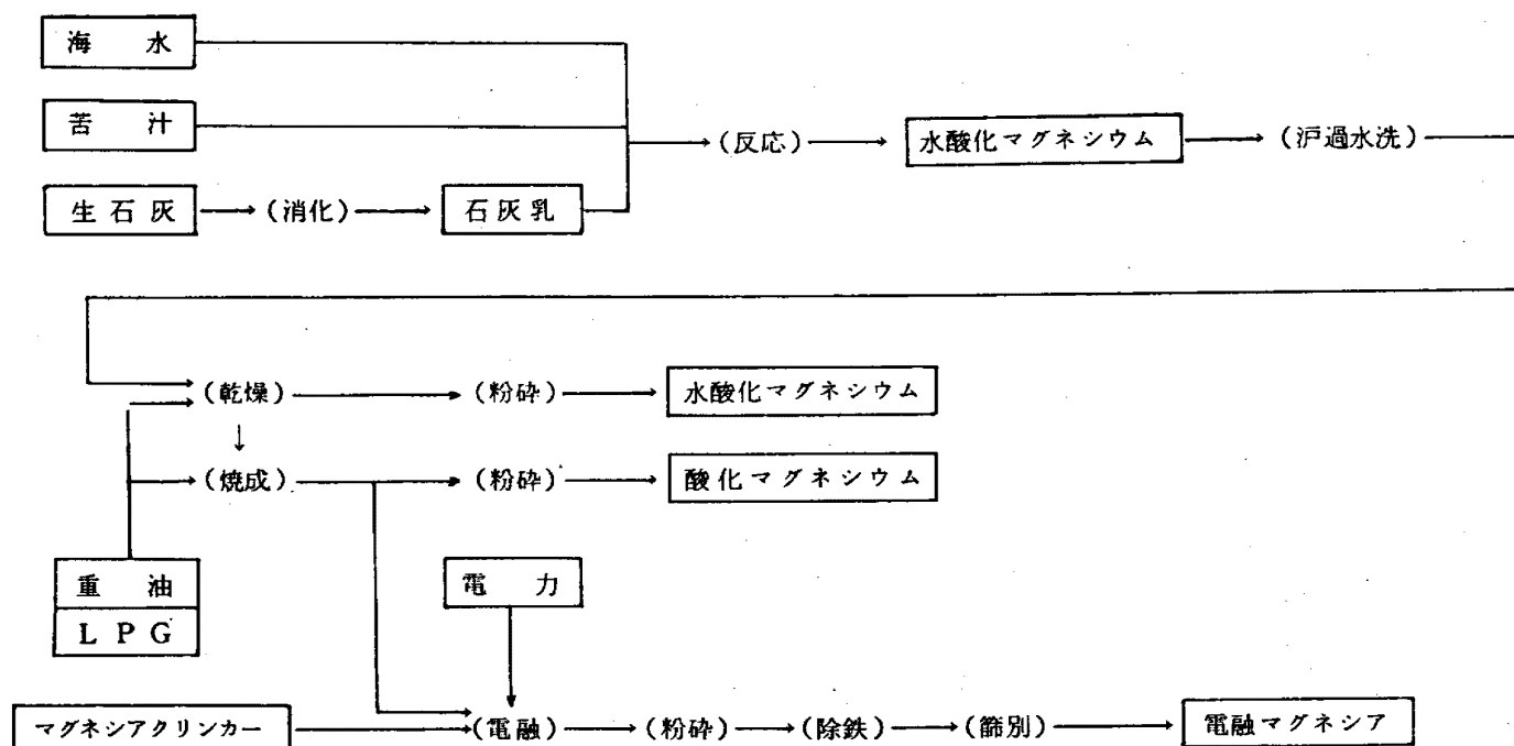
電融マグネシア、酸化マグネシウム、水酸化マグネシウムの製造工程図
