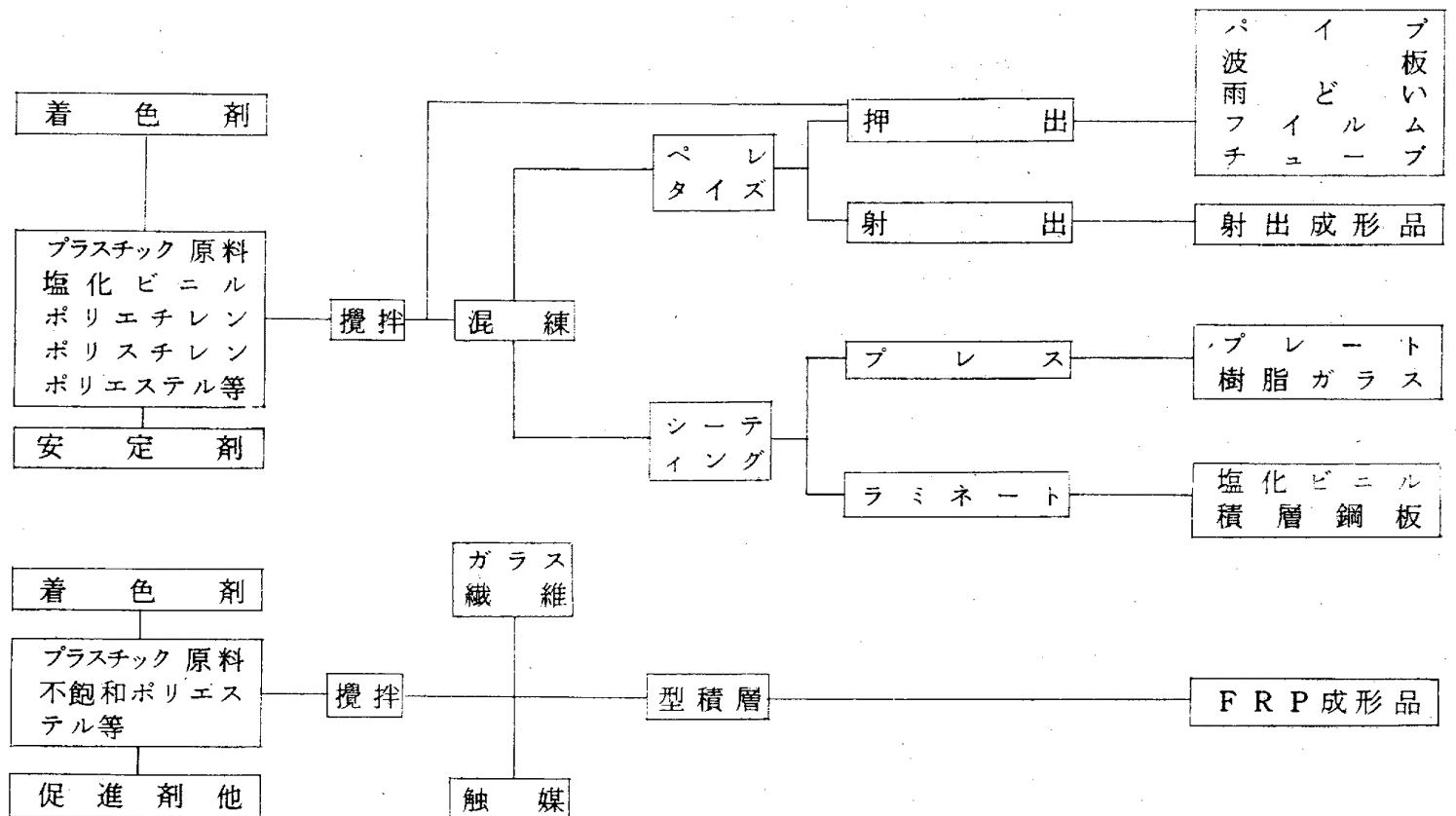
主要製品製造工程図表
