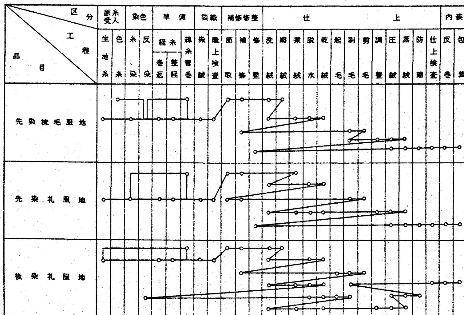
主 要 製 品 の 製 造 工 程 図
