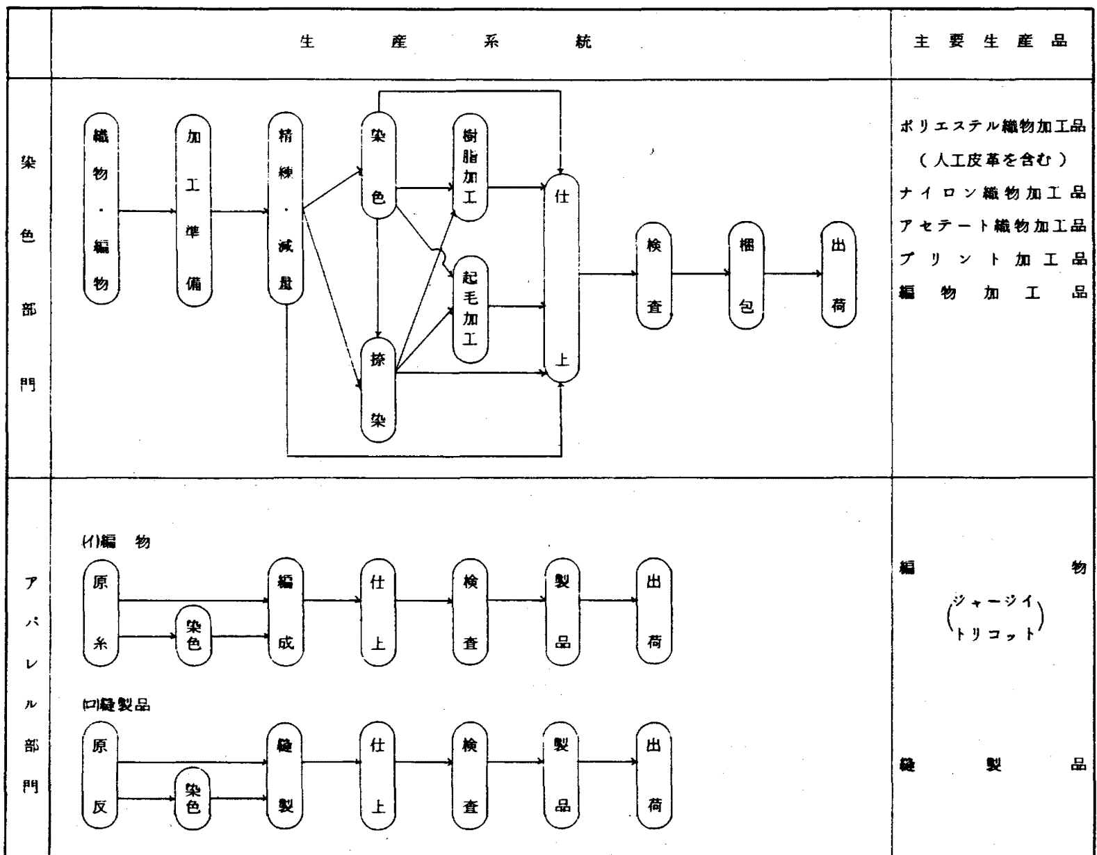
生産系統図
